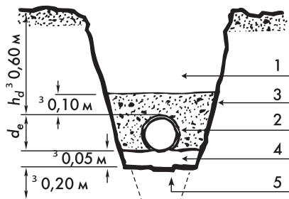
Рис. 6.1 Конструкция траншеи
